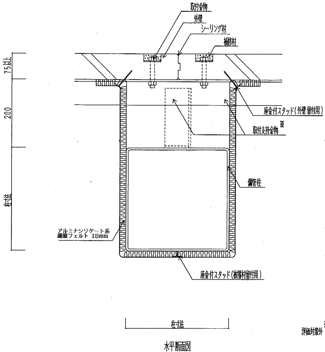
図1 構造説明図(角形鋼管柱仕様)
